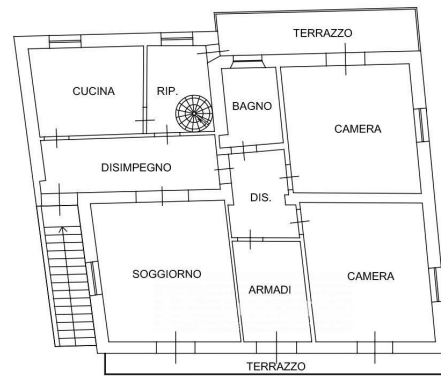
PIANO PRIMO H=3.00
